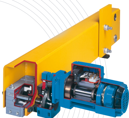
Kranfahrwerk mit Fahrtrieb
